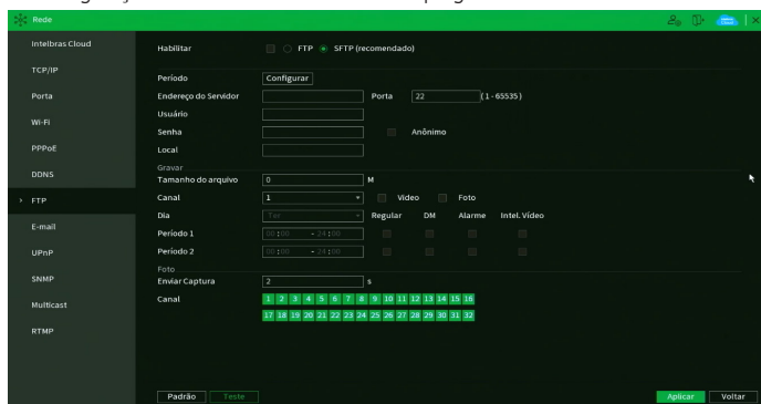
Menu FTP
