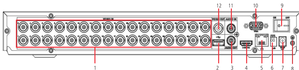
Panel posterior
